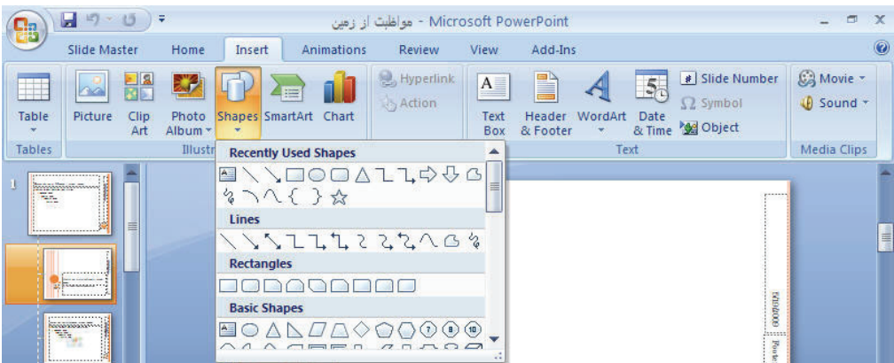
شکل ۴-۷) انتخاب شکل
