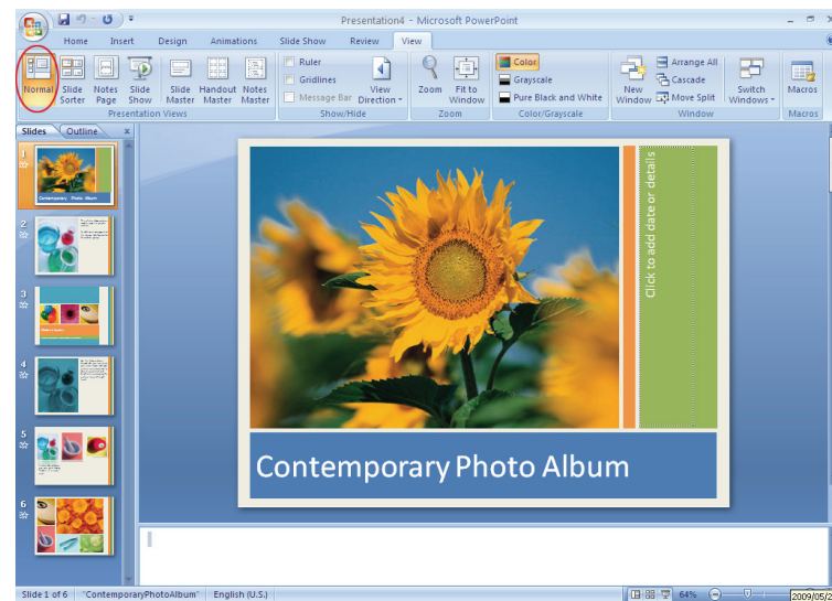
شکل ۱۰-۲) نمای Normal
